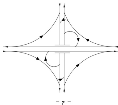
شکل ۹-۹- نمونه طرح‌های ورودی و خروجی تبادلهای نیمه‌شبه‌دوری
