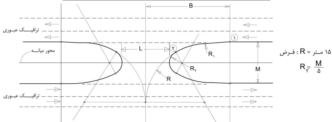
شکل ۸-۴- طرح بیش از حداقل برای بریدگی‌های میانه (انتهای سرفشنگی)
