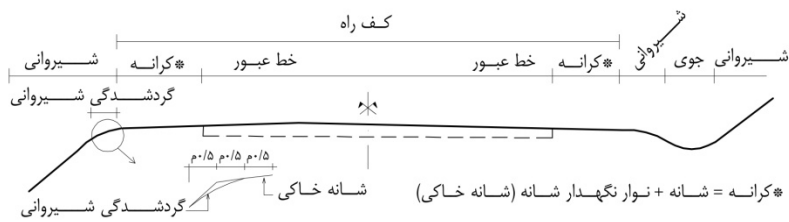
شکل ۶-۲- اجزای نیمرخ عرضی در راه‌های دو خطه و چهار خطه
