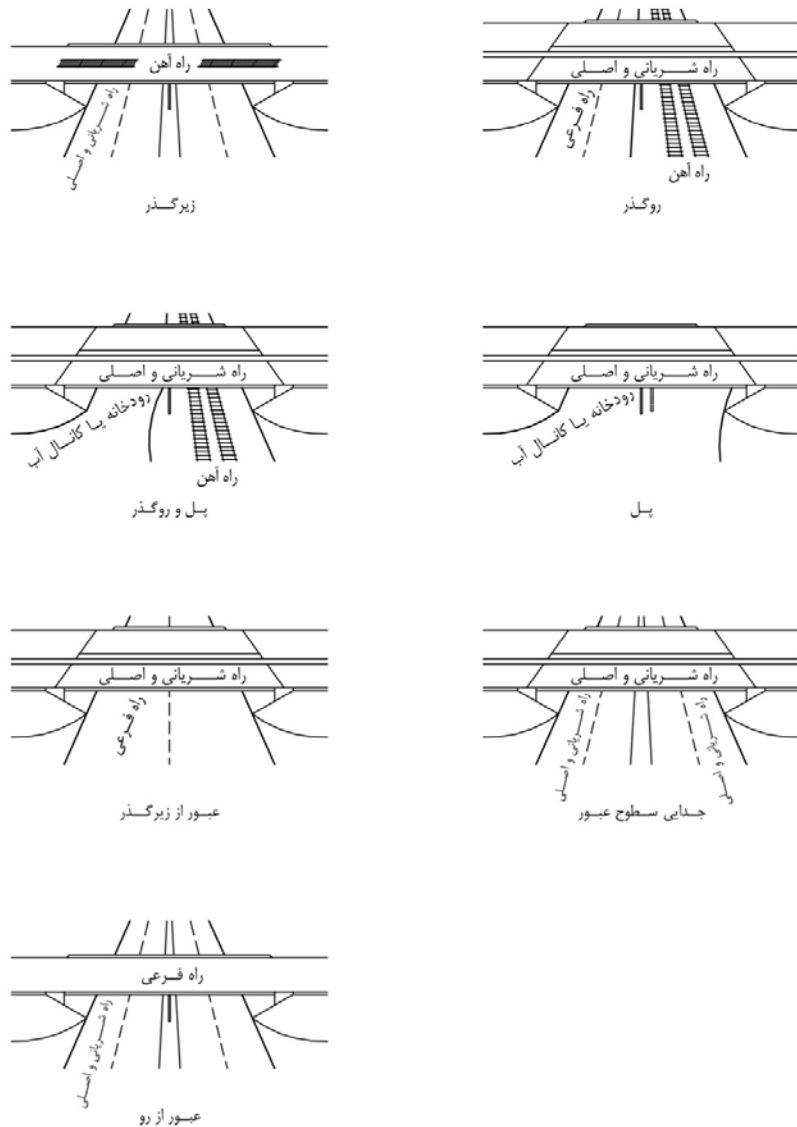
شکل ۹-۱۵- انواع زیرگذر و روگذر
