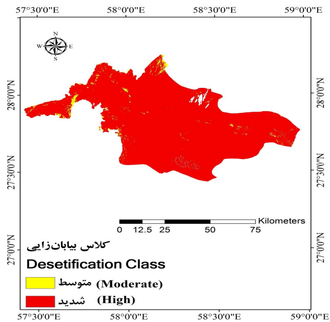
شکل ۴- نقشه پتانسیل بیابان‌زایی با استفاده از مدل IMDPA و با تأکید بر معیار فرسایش.
