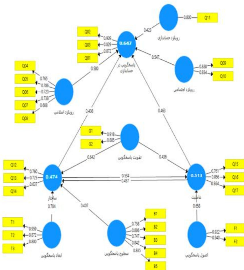
شکل ۱. مدل پژوهش در حالت تخمین ضرایب استاندارد
