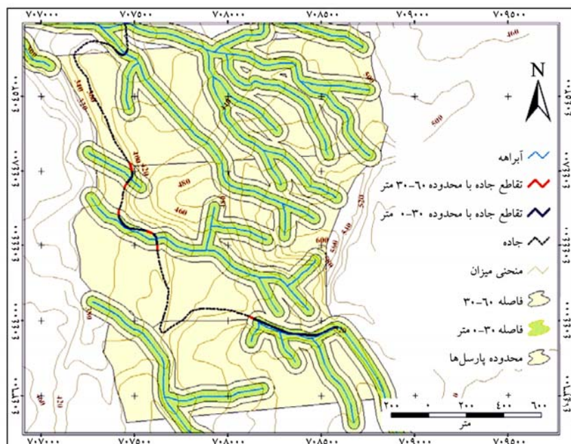
شکل ۱- نقشه شبکه زه‌کشی، جاده‌های جنگلی و بافرهای تهیه شده بین جاده و آبراه در محیط GIS.
