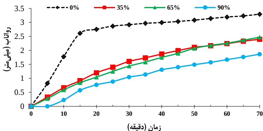
شکل ۲- نمودار تغییرات زمانی ارتفاع رواناب در درصد‌های مختلف پوشش گیاهی
