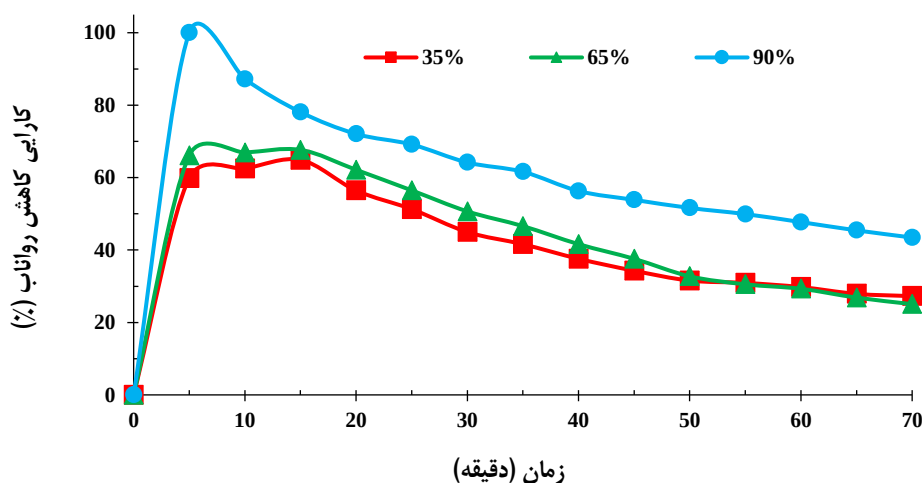
شکل ۳- نمودار تغییرات زمانی کارایی کاهش رواناب در درصد‌های مختلف پوشش گیاهی
