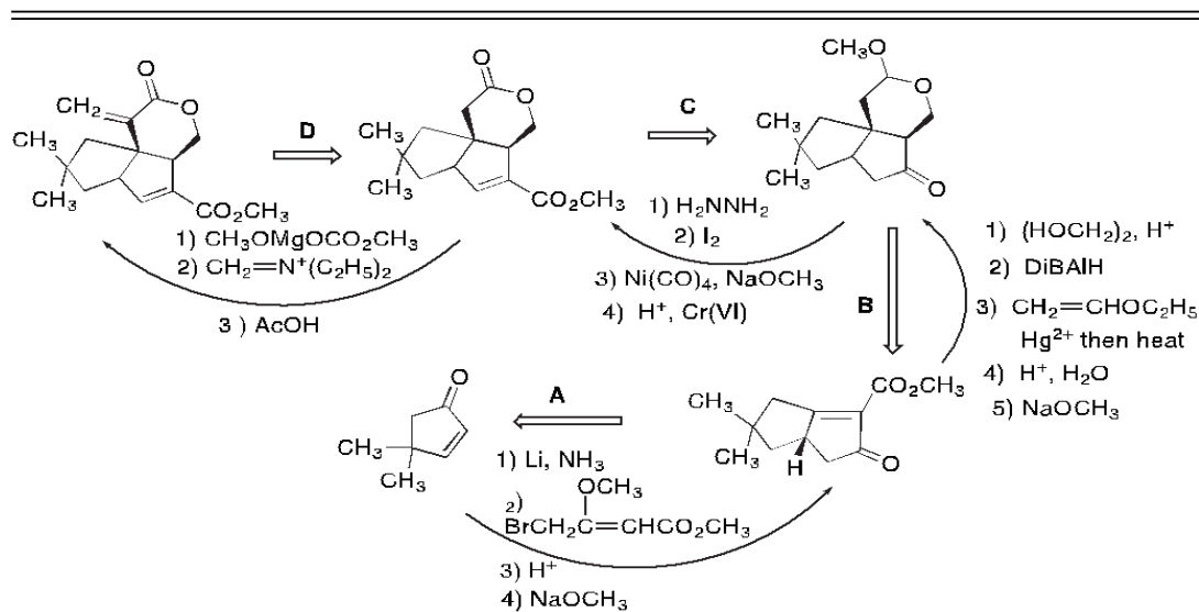
Scheme 13.P9c-2. Pentalenolactone E Synthesis: L. A. Paquette, G. D. Annis, and H. Schostarez a
