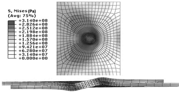
شکل 13 کانتور تنش فون مایز برای قطر ناگت 6 میلی متر تحت نیروی 5000 نیوتن
