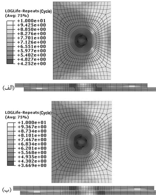
شکل 16 تحلیل خستگی برای قطر ناگت 6 میلی متر تحت نیروی 5000 نیوتن (الف)
